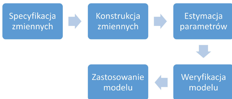
Rysunek 1. Procedura ekonometryczna.
