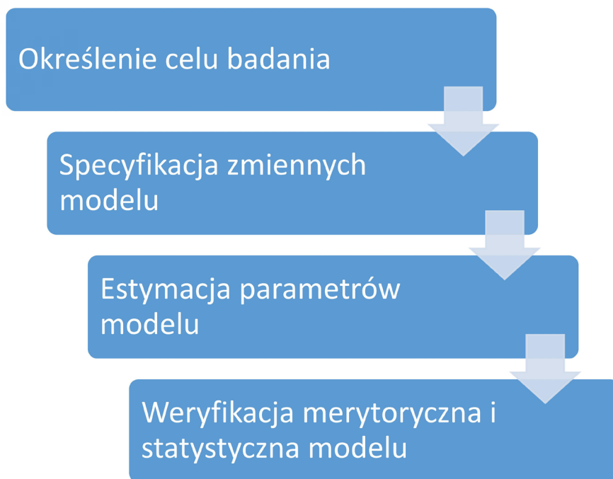
Rysunek 4. Etapy budowy modelu ekonometrycznego.
