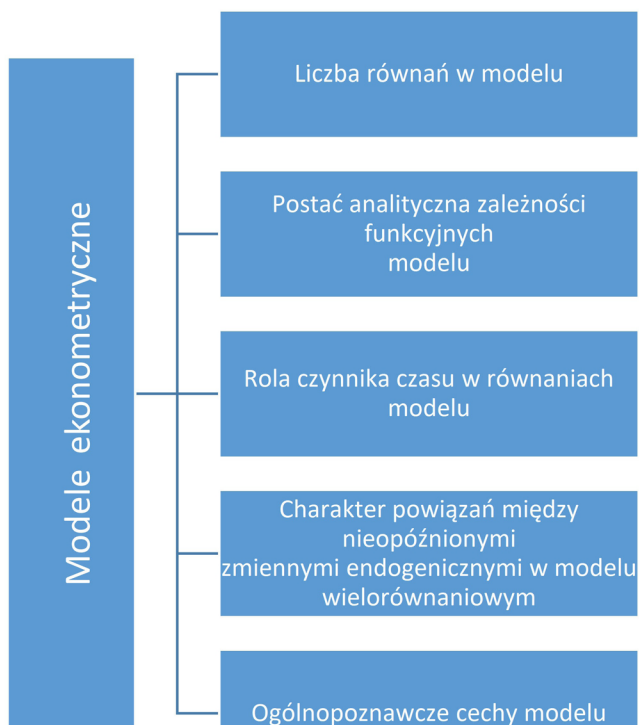
Rysunek 3. Klasyfikacja modeli ekonometrycznych.
