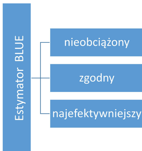
Rysunek 22. Własności estymatora BLUE.
