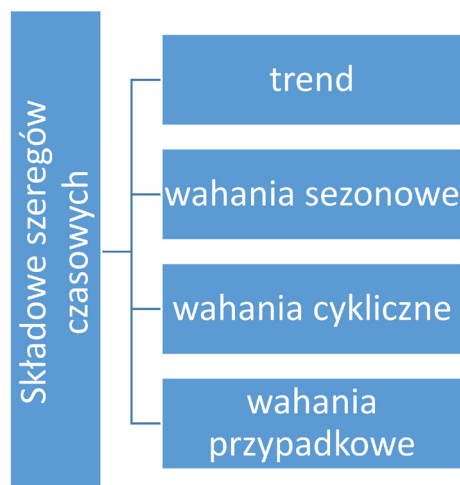
Rysunek 42. Składowe szeregów czasowych.
