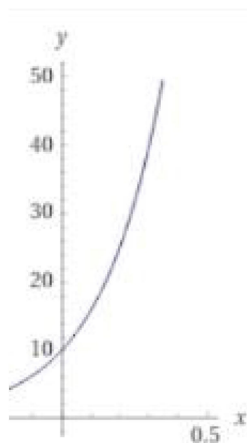
Rysunek 12. Funkcja wykładnicza Y = 10^{aX+c} dla a > 0 .
