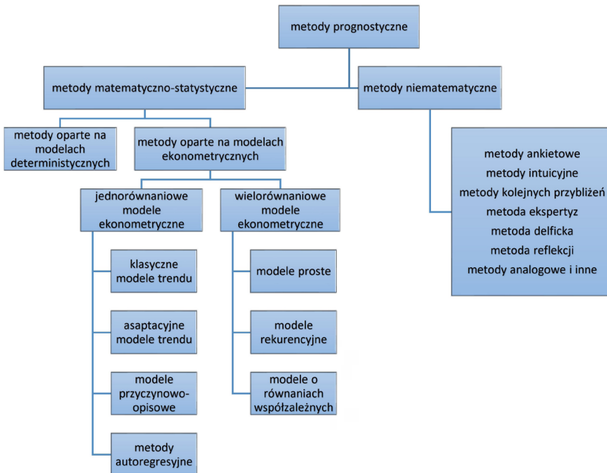
Rysunek 37. Metody prognozowania.
