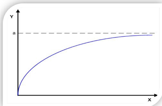
Rysunek 14. Wykres funkcji Törnquista I typu.
