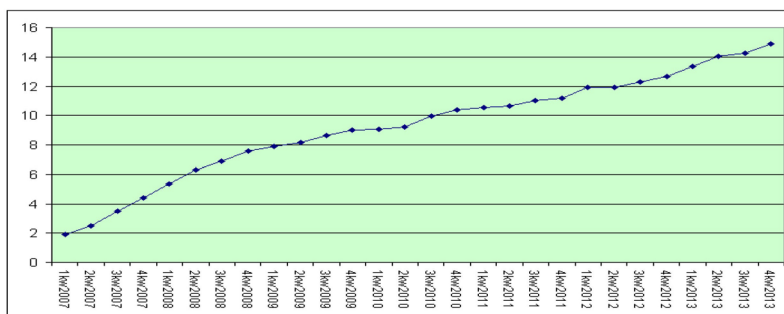
Rysunek 40. Trend.
