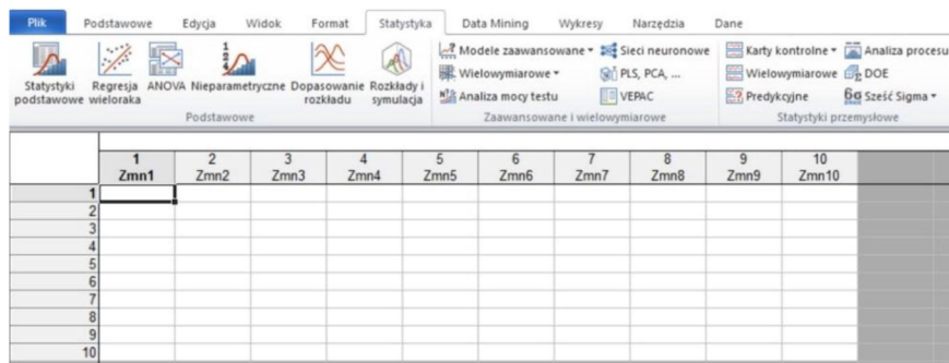
Rysunek 18. Interfejs programu Statistica.
