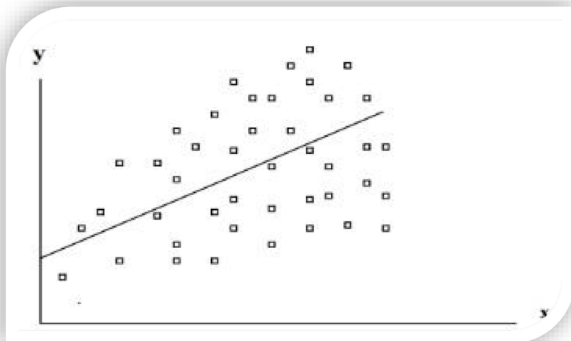
Rysunek 30. Heteroskedastyczność.
