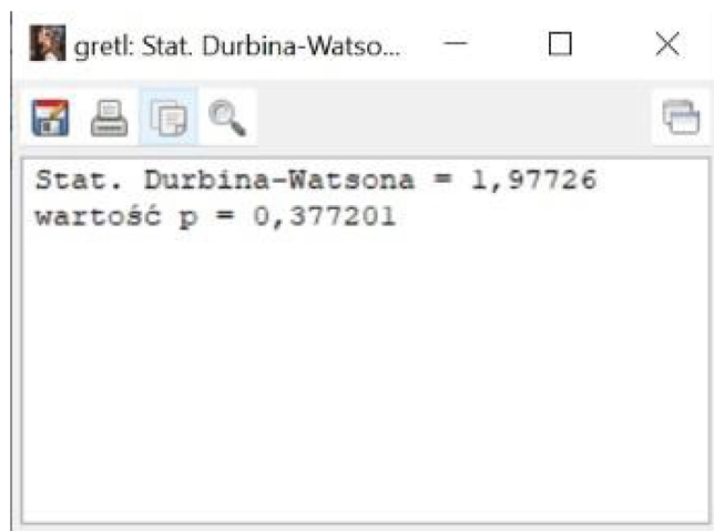
Rysunek 28. Wyniki testu Durбина-Watsona w programie Gretl.
