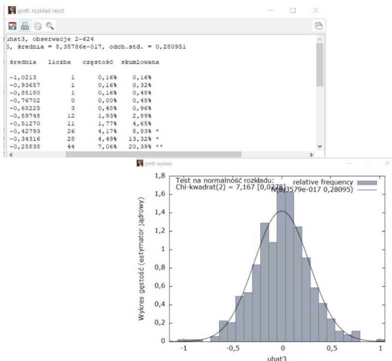
Rysunek 27. Wyniki testu oceny normalności w programie Gretl.
