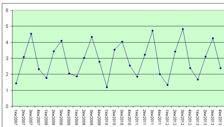
Rysunek 41. Składowa okresowa.
