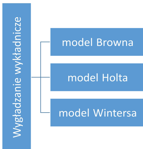
Rysunek 43. Modele wygładzania wykładniczego.
