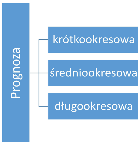
Rysunek 34. Rodzaje prognoz ze względu na okres prognozy.
