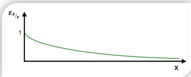
Rysunek 15. Wykres elastyczności dla funkcji Törnquista I typu.
