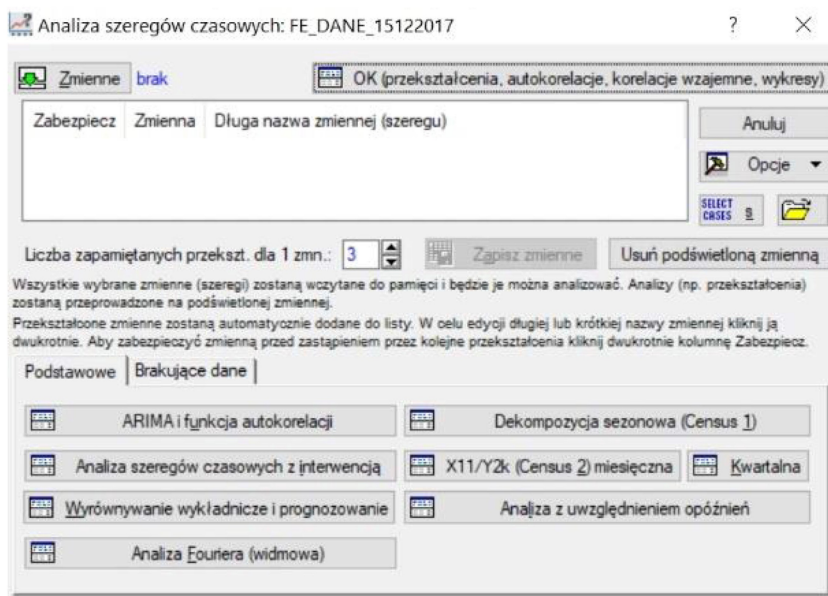
Rysunek 19. Moduł Analiza szeregów czasowych.
