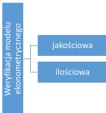
Rysunek 24. Weryfikacja modelu ekonometrycznego.
