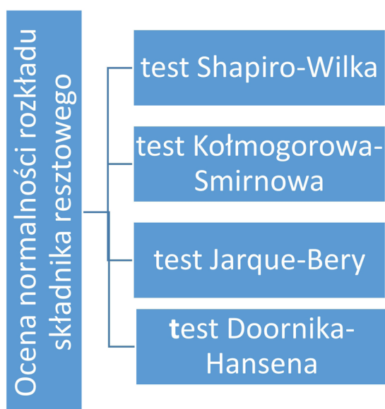
Rysunek 26. Testy oceny normalności rozkładu składnika resztowego.
