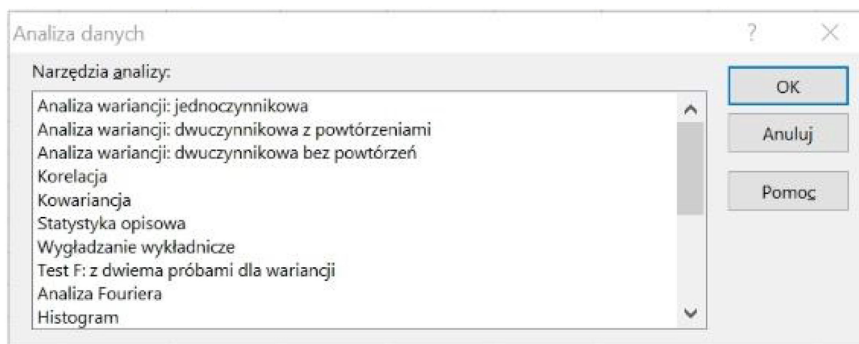
Rysunek 17. Dostępne funkcje Analizy danych.
