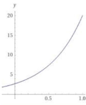
Rysunek 10. Funkcja wykładnicza Y = e^{aX+c} dla a > 0 .
