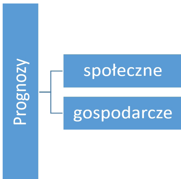
Rysunek 36. Prognozy ze względu na rodzaj prognozowanego zjawiska.
