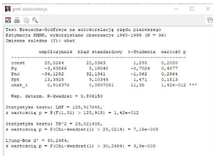
Rysunek 29. Wyniki testu Breuscha-Godfrey w programie Gretl.
