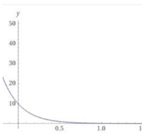
Rysunek 13. Funkcja wykładnicza Y = 10^{aX+c} dla a < 0 .
