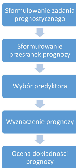
Rysunek 38. Etapy prognozowania ekonometrycznego.
