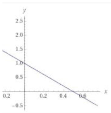
Rysunek 9. Funkcja liniowa dla a < 0 .
