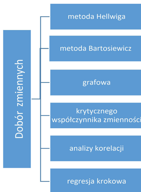
Rysunek 5. Metody doboru zmiennych objaśniających.
