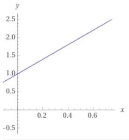
Rysunek 8. Funkcja liniowa dla a > 0 .
