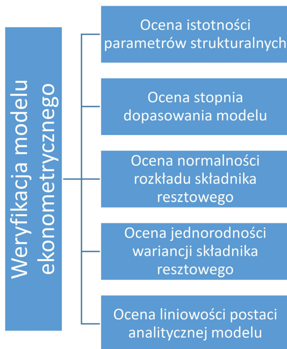
Rysunek 25. Etapy weryfikacji modelu ekonometrycznego.
