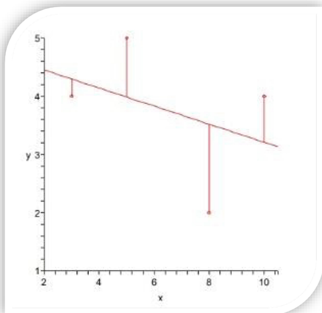
Rysunek 21. Metoda najmniejszych kwadratów.
