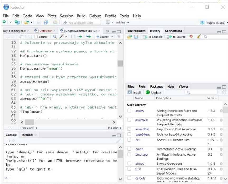
Rysunek 20. Okno RStudio.
