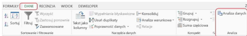
Rysunek 16. Moduł Analiza danych pakietu Excel.
