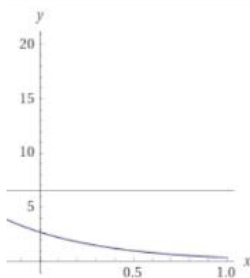
Rysunek 11. Funkcja wykładnicza Y = e^{aX+c} dla a < 0 .
