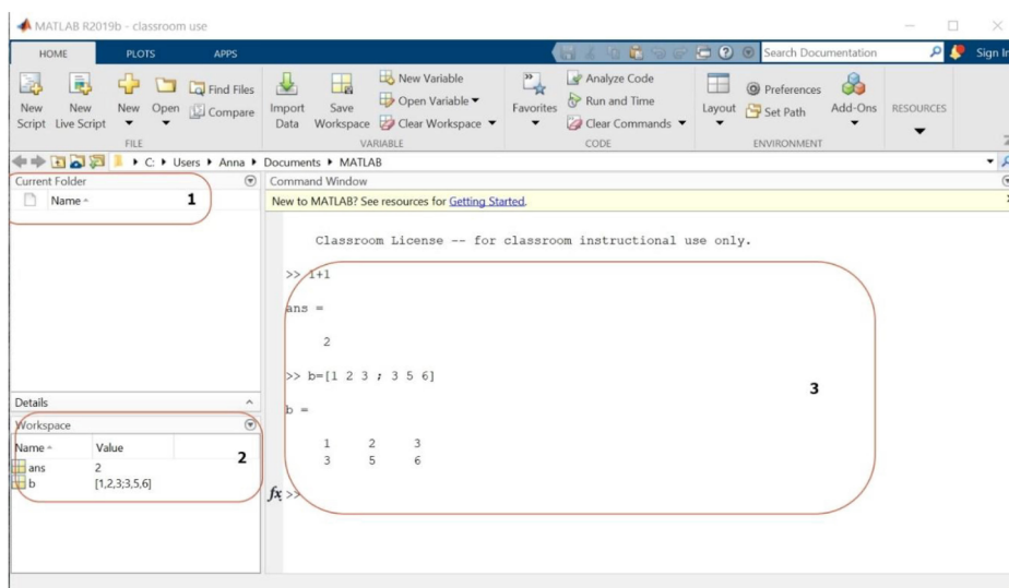
Rysunek 2. Główne okno Matlaba.
