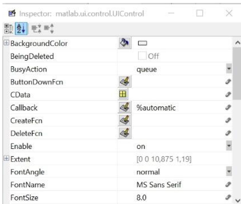
Rysunek 18. Okno inspektora właściwości obiektu ( Prosperity inspector ).
