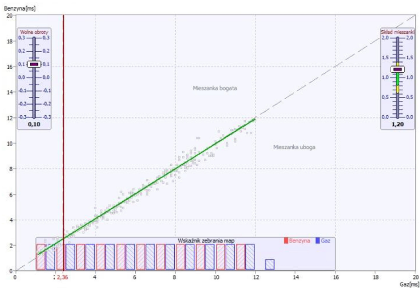
Rys. 5.6. Okno Mapa-> Mapa 2D software.
