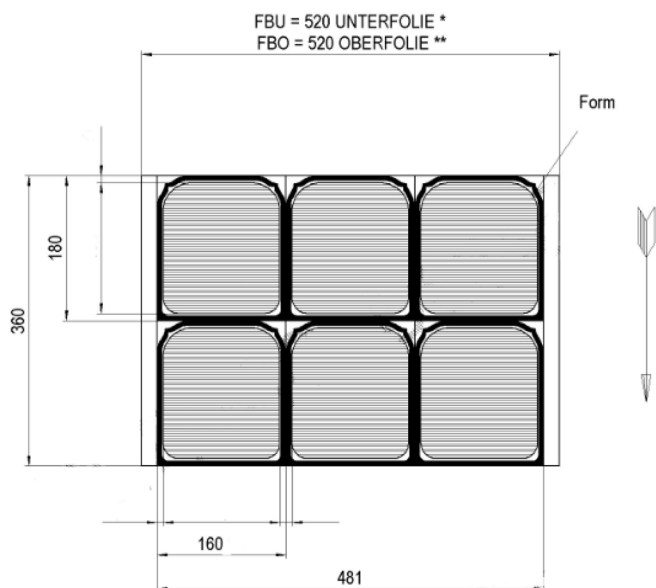
Rys. 2.1. Format opakowań.
