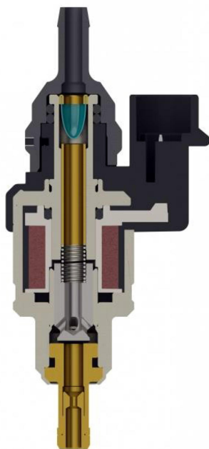
Rys. 5.21. Widok w przekroju wtryskiwacza gazowego Barracuda firmy Alex [58].
