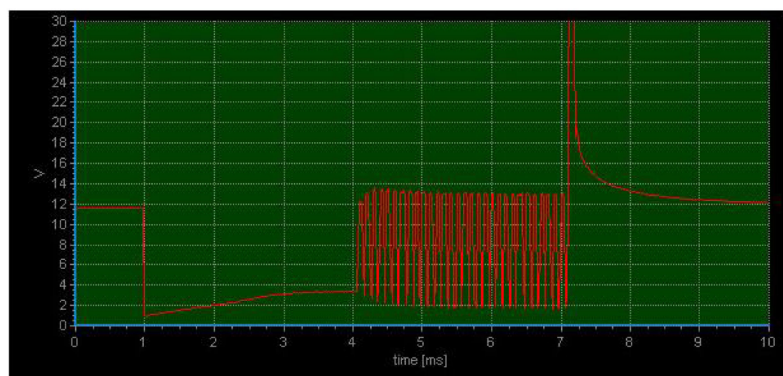
Rys. 5.10. Przykładowy poprawny przebieg napięcia otwarcia wtryskiwacza gazowego.
