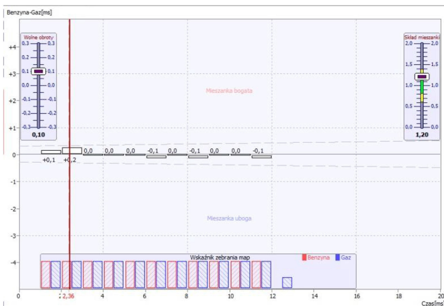
Rys. 5.8. Odchyłki w składzie mieszanki paliwowo-gazowej w stosunku do paliwowo-benzynowej.
