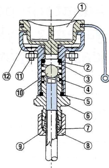
Rys. 5.16. Przekrój przez wlew paliwa [20]:
