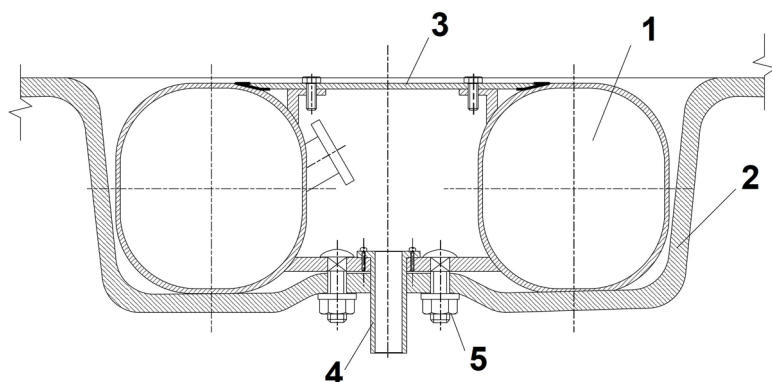
Rys. 5.13. Mocowanie zbiornika toroidalnego wewnętrznego:
