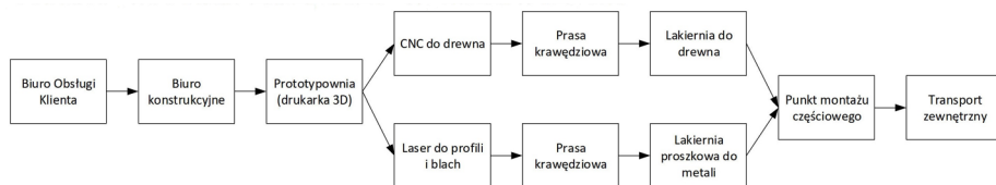
Rys. 1.3. Linia Szybkiego Prototypowania Systemów Ekspozycyjnych JBM.
