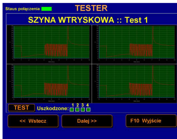
Rys. 5.9. Okno testu sygnałów otwierających wszystkie wtryskiwacze.
