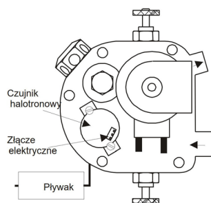
Rys. a) Zawór Lovato prawy
