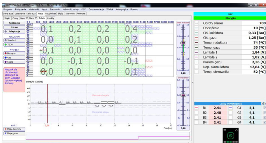
Rys. 5.39. Okno kalibracji systemu wtrysku LPG.
