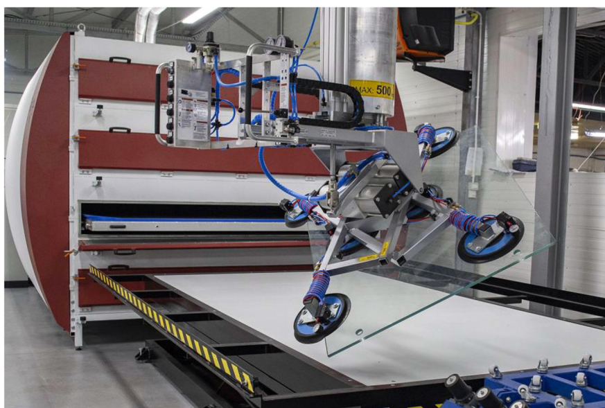
Rys. 4.6. Wygląd linii technologicznej podczas przenoszenia szkła.
