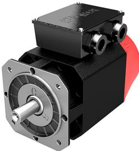
Rys. 2.7. Serwosilnik PMSM do maszyny CNC [63].
