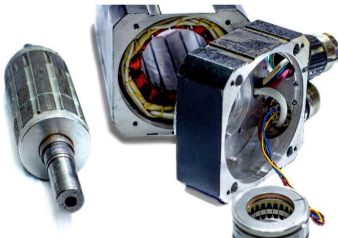
Rys. 2.8. Rozmontowany serwosilnik PMSM do maszyny CNC [64].
