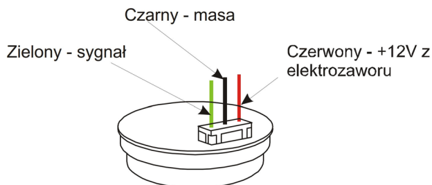
Rys. 5.17. Widok czujnika SPW01.
