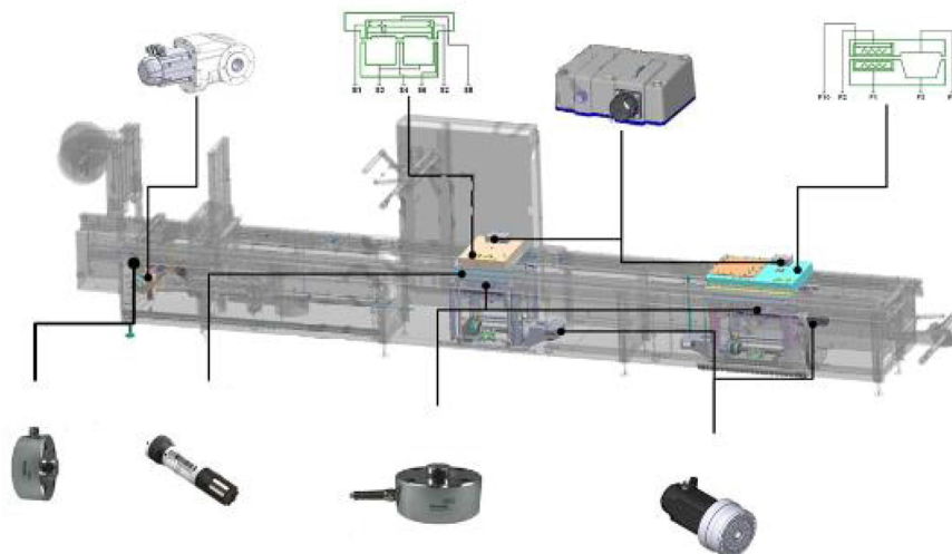
Rys. 4.8. Przykład rozmieszczenia czujników w maszynie rolowej [75].
