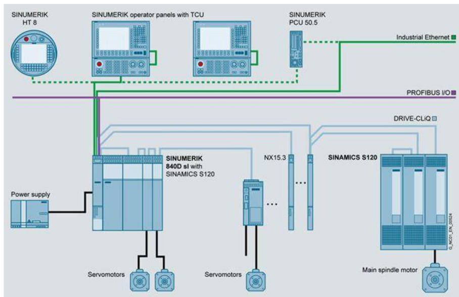
Rys. 2.16. Komponenty i sposób sterowania nimi w SINUMERIK [65].
