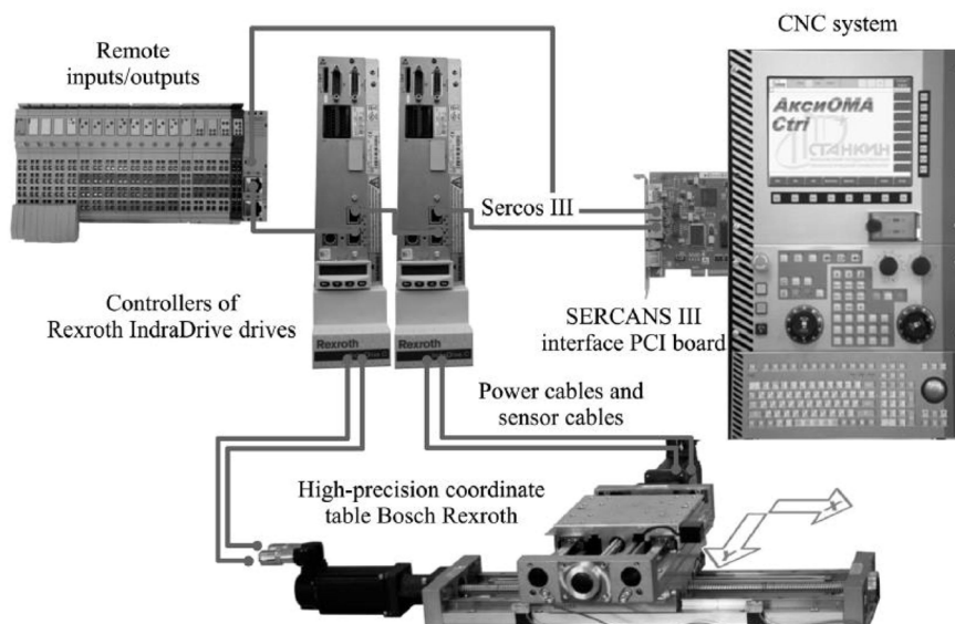
Rys. 2.10. Sterowanie odcinkowe stołem frezerskim [22].
