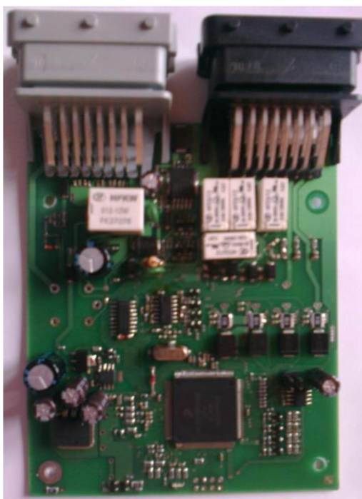
Rys. 5.3. Płytką drukowaną elektronicznej jednostki sterującej wtryskiem LPG – góra.
