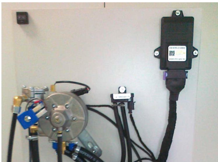
Rys. 5.26. Rozmieszczenie ECU.
