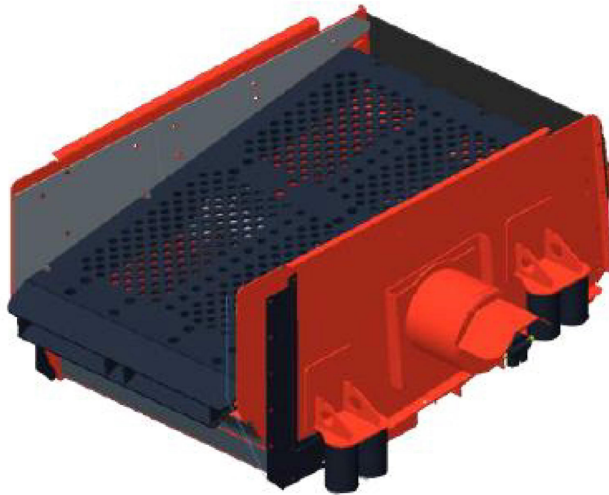
Rys. 3.5. Odsiewacz wstępny dwupokładowy [76].
