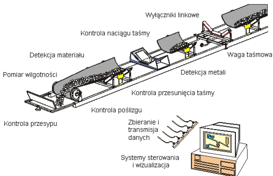
Rys. 3.20. Opcjonalne systemy automatyki [78].
