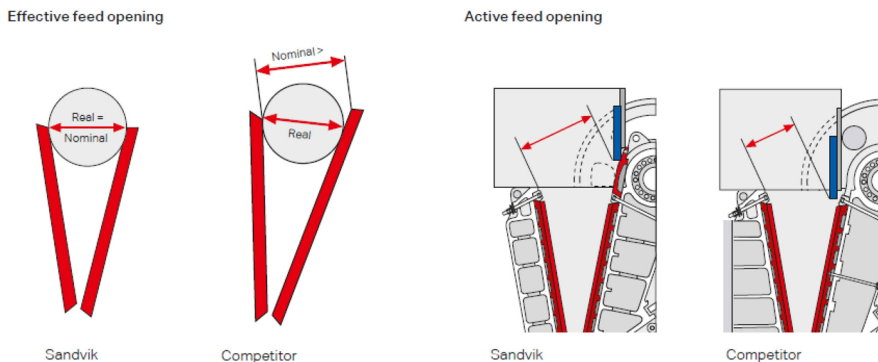
Rys. 3.2. Otwór zasypowy w kruszarce Sandvik [76].
