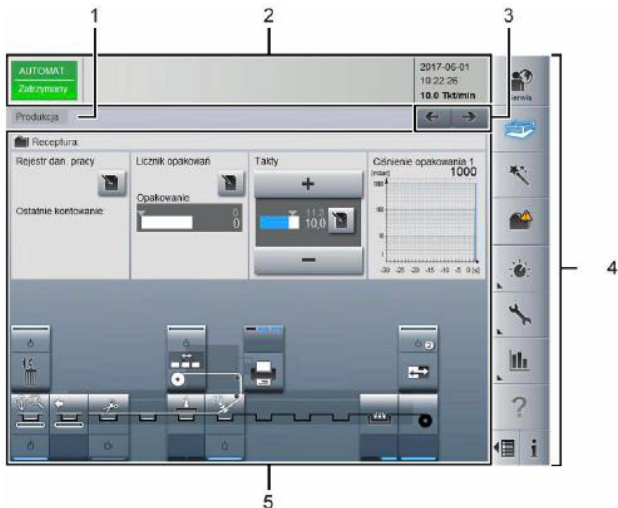
Rys. 4.7. Wyświetlacz w maszynie rolowej [75].
