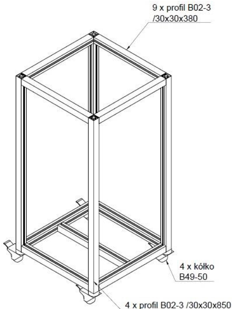
Rys. 5.24. Rysunek złożeniowy wykonawczy wózka jeźdnego.
