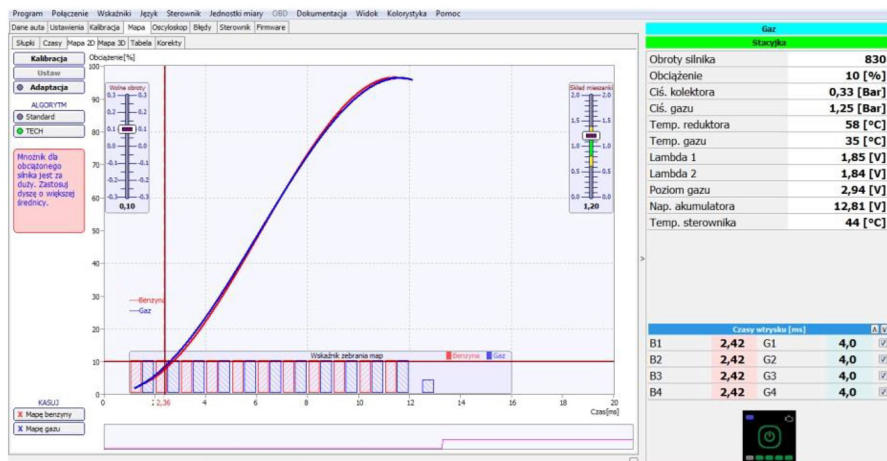
Rys. 5.5. Okno Mapa-> Mapa 2D software.
