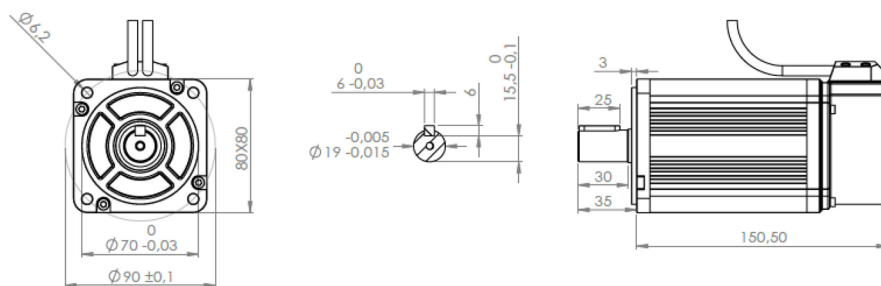
Rys. 2.13. Główne wymiary serwosilnika [67].
