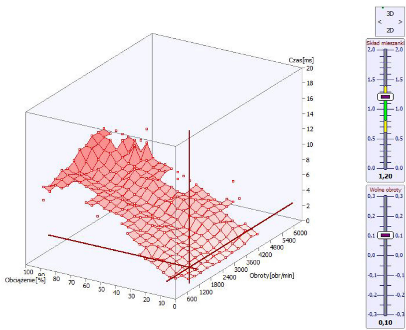
Rys. 5.7. Okno Mapa-> Mapa 3D software.
