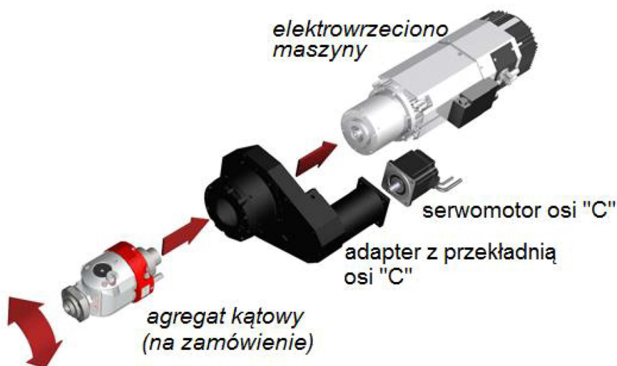
Rys. 2.9. 4 oś C – adapter do agregatu na wrzeciono HSD ze stożkiem ISO 30 [62].
