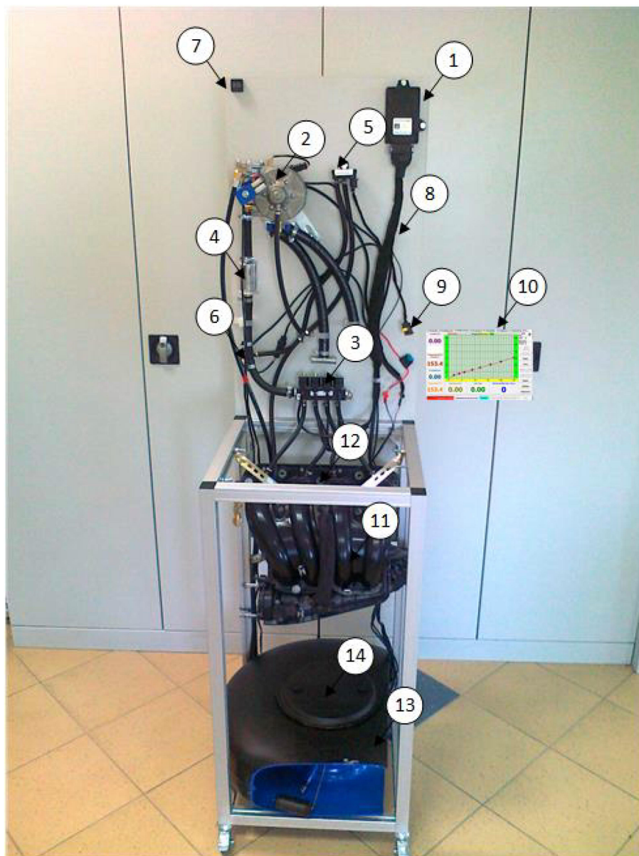
Rys. 5.32. Specyfikacja elementów interaktywnego stanowiska systemu sekwencyjnego wtrysku gazu LPG.
