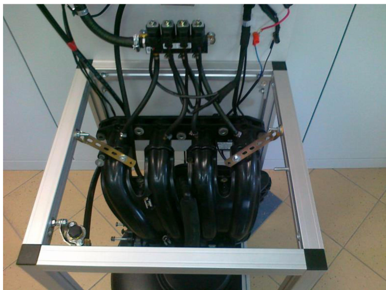
Rys. 5.29. Rozmieszczenie kolektora dolotowego i wtryskiwaczy.
