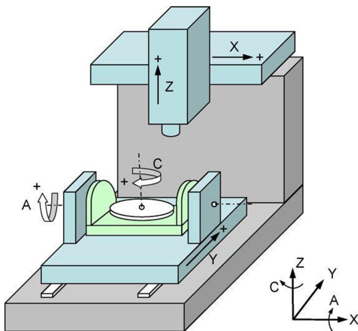
Rys. 2.1. Schemat budowy obrabiarki sterowanej numerycznie CNC o pięciu osiach [12].
