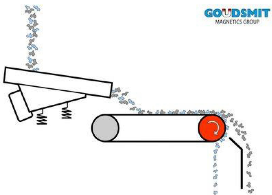
Rys. 3.16. Zasada działania bębnowego separatora magnetycznego.
