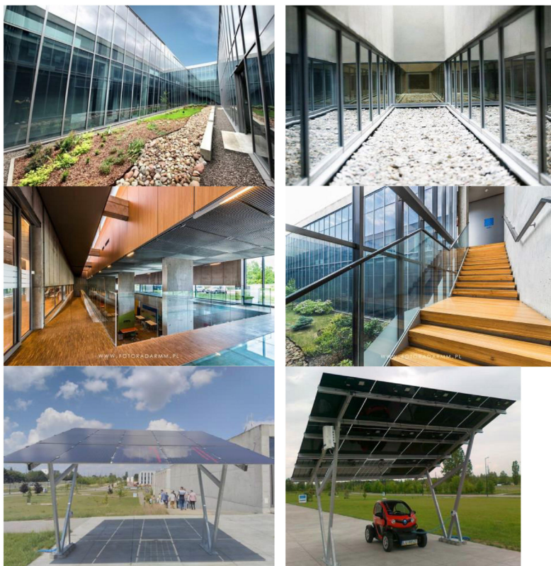
Rys. 4.2. Zastosowanie szkła w budynku Lubelskiego Parku Naukowo-Technologicznego [27].
