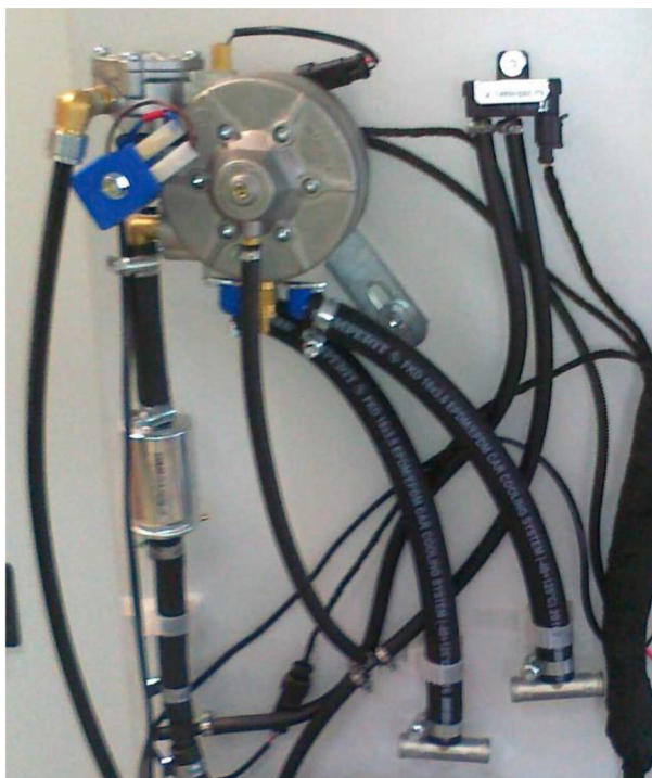
Rys. 5.27. Rozmieszczenie reduktora i czujnika ciśnienia.
