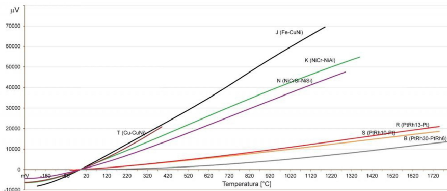
Rys. 3.25. Charakterystyki termopar [78].
