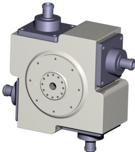
Rys. 2.3 Rewolwerowa głowica CNC P4MAN [59].
