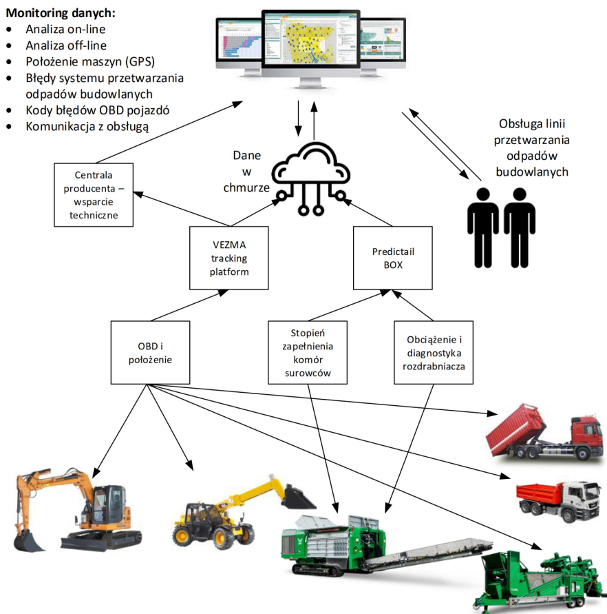
Rys. 3.1. Kompletny system zarządczy mobilnej linii przetwarzania odpadów budowlanych.
