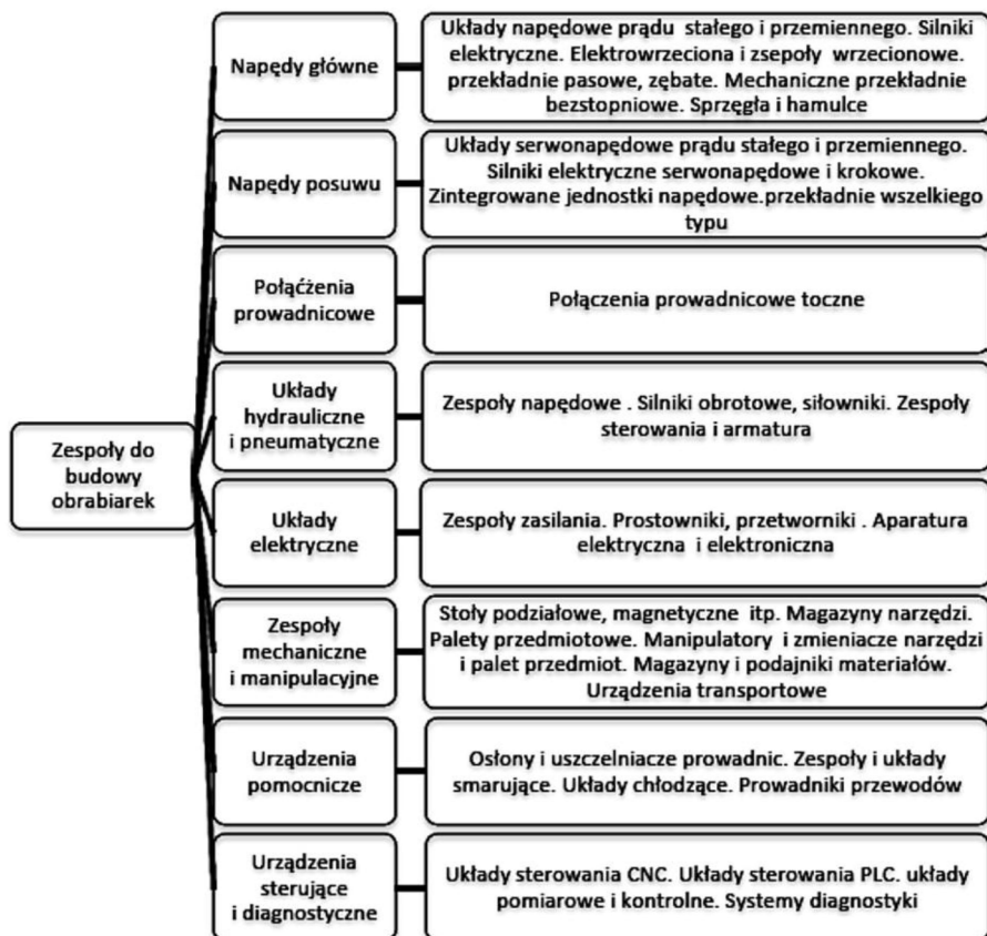
Rys. 2.2. Podstawowe zespoły funkcjonalne obrabiarek CNC [15].
