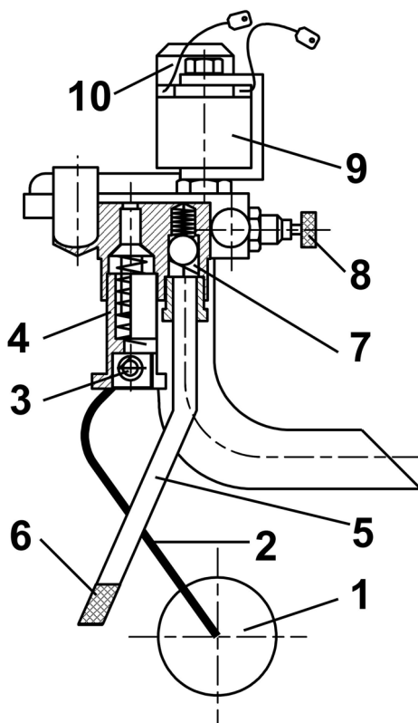
Rys. 5.15. Wielozawór [20]:
