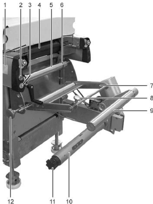
Rys. 4.2. Układ podawania folii dolnej w maszynie rolowej do pakowania próżniowego [75].
