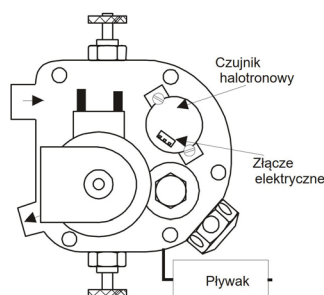
Rys. b) Zawór Lovato lewy
